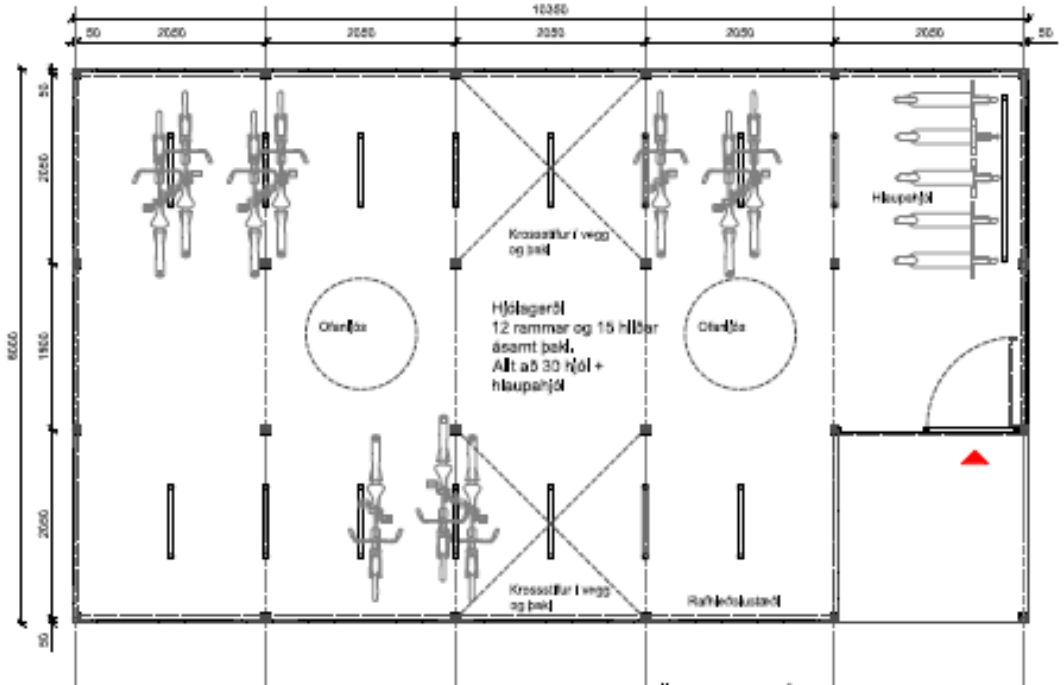
GRUNNMYND - LOKAÐ TVÖFALT SKÝLI mkv. 1:50
