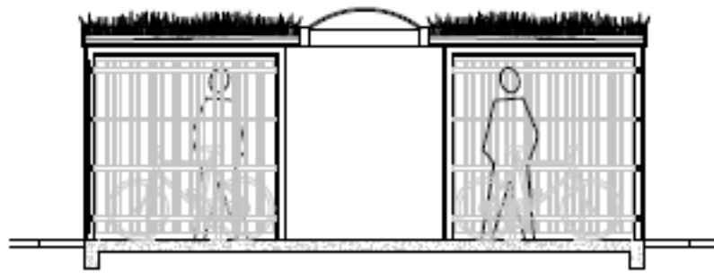
SNEIÐING 2 - LOKUÐ MIÐJA mkv. 1:50
