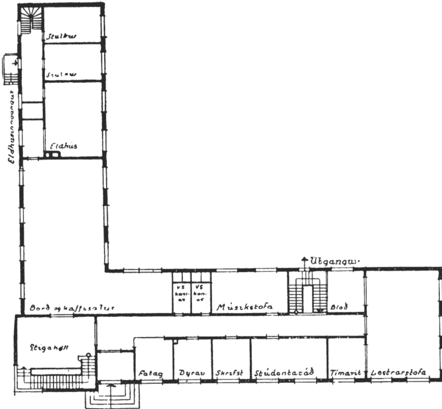
Tillöguuppráttur að stúdentagarði, 1930, eftir Einar Sveinsson og Gunnlaug Halldórsson. (Úr Stúdentblaði 1930.)
